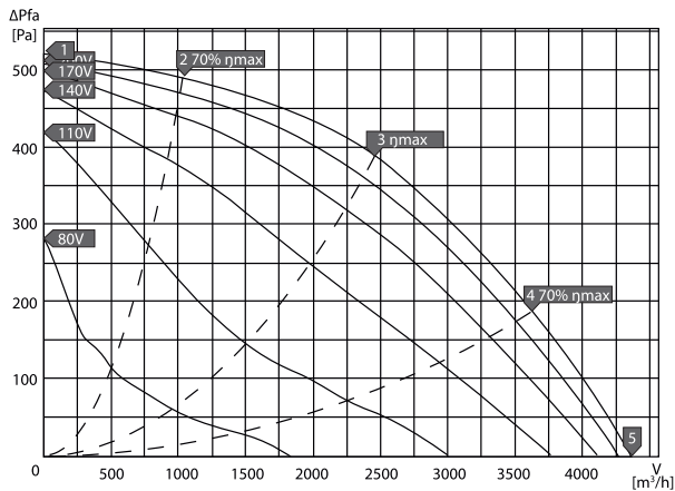
KCF-N 400 E4 20
