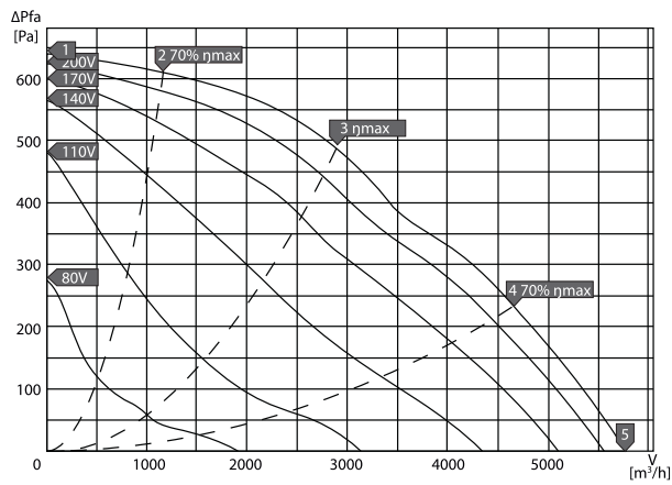
KCF-N 450 E4 20
