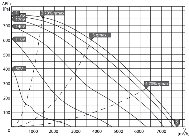
KCF-N 500 E4 20
