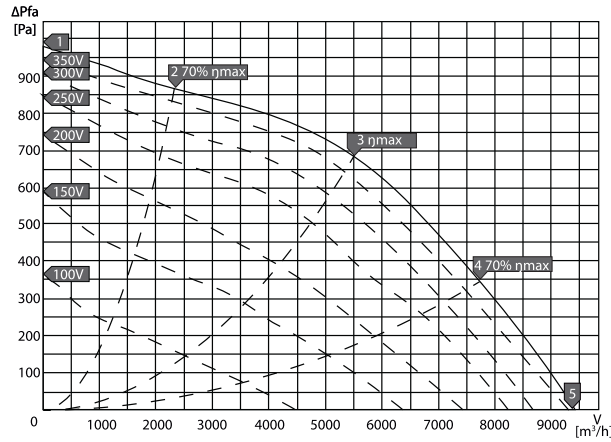
KCF-N 560 D4
